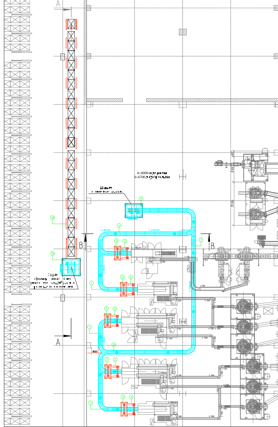
План 1-го этажа
