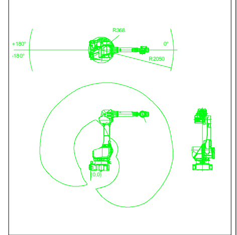
Робот-манипулятор
